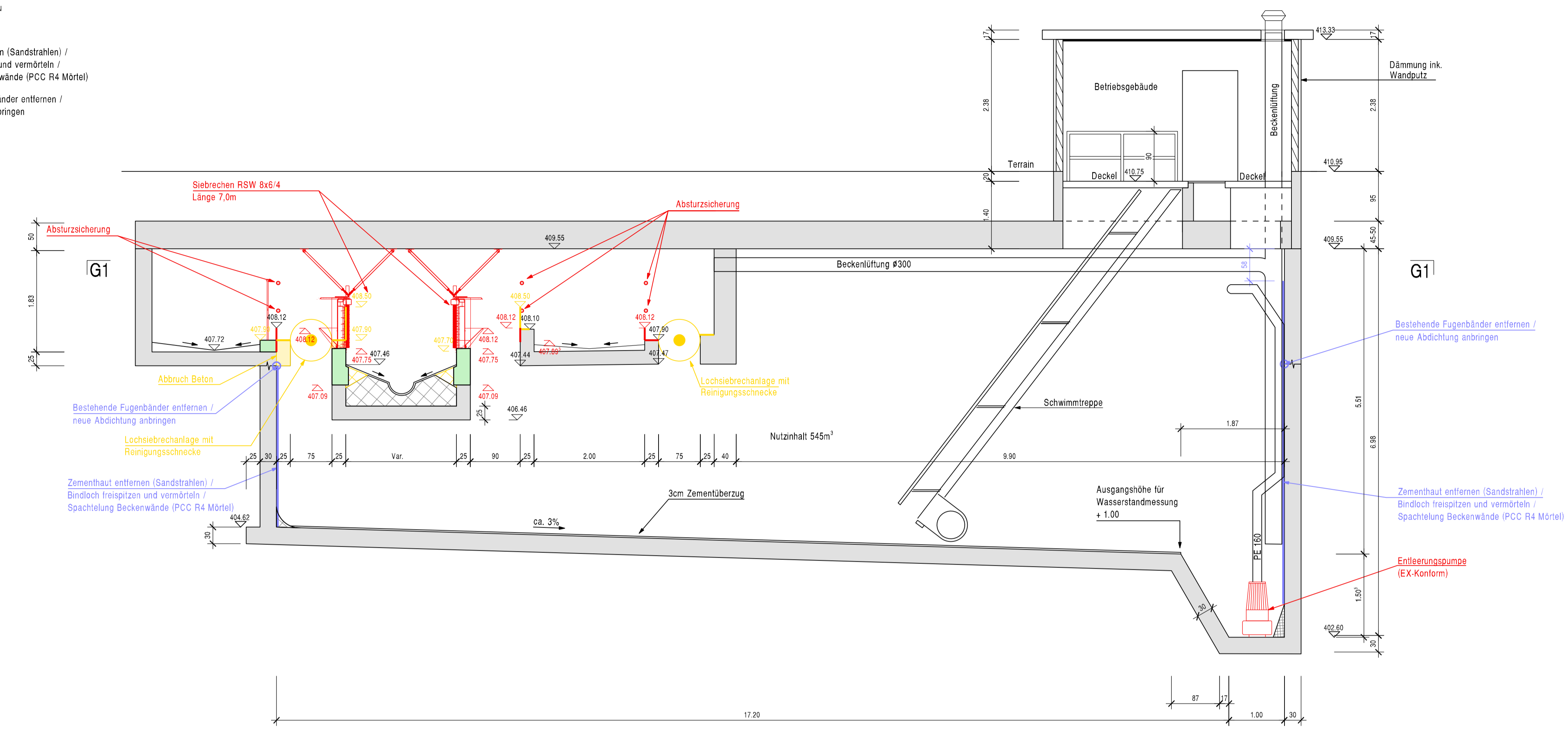
Schnitt A-A 1:50
