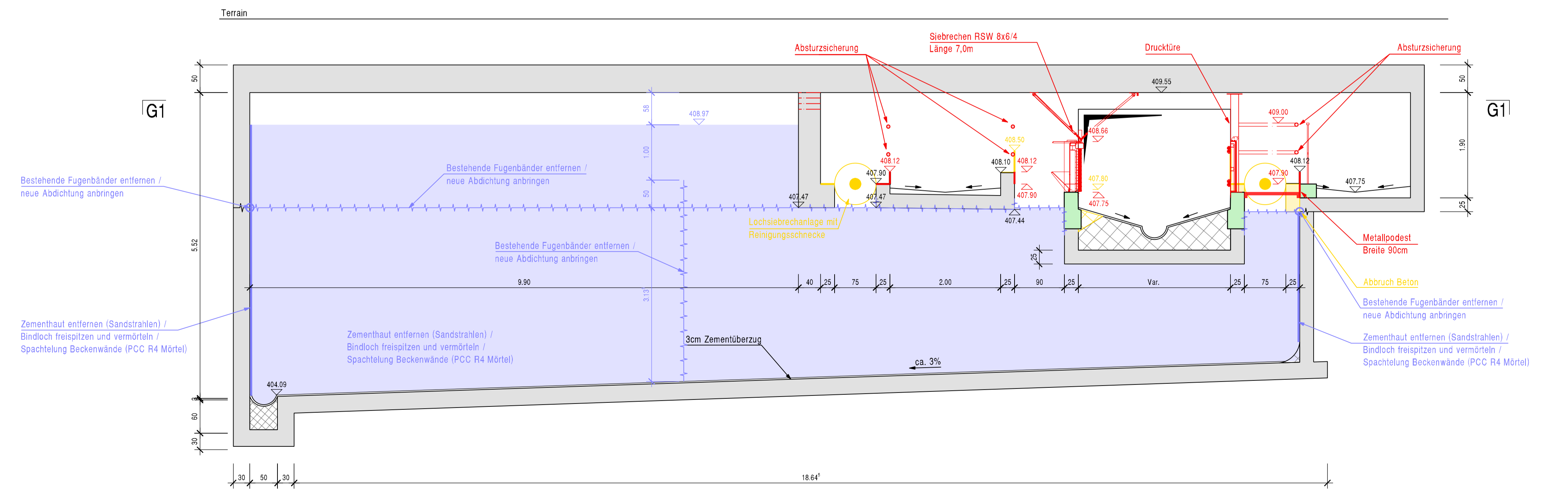
Schnitt D-D 1:50
