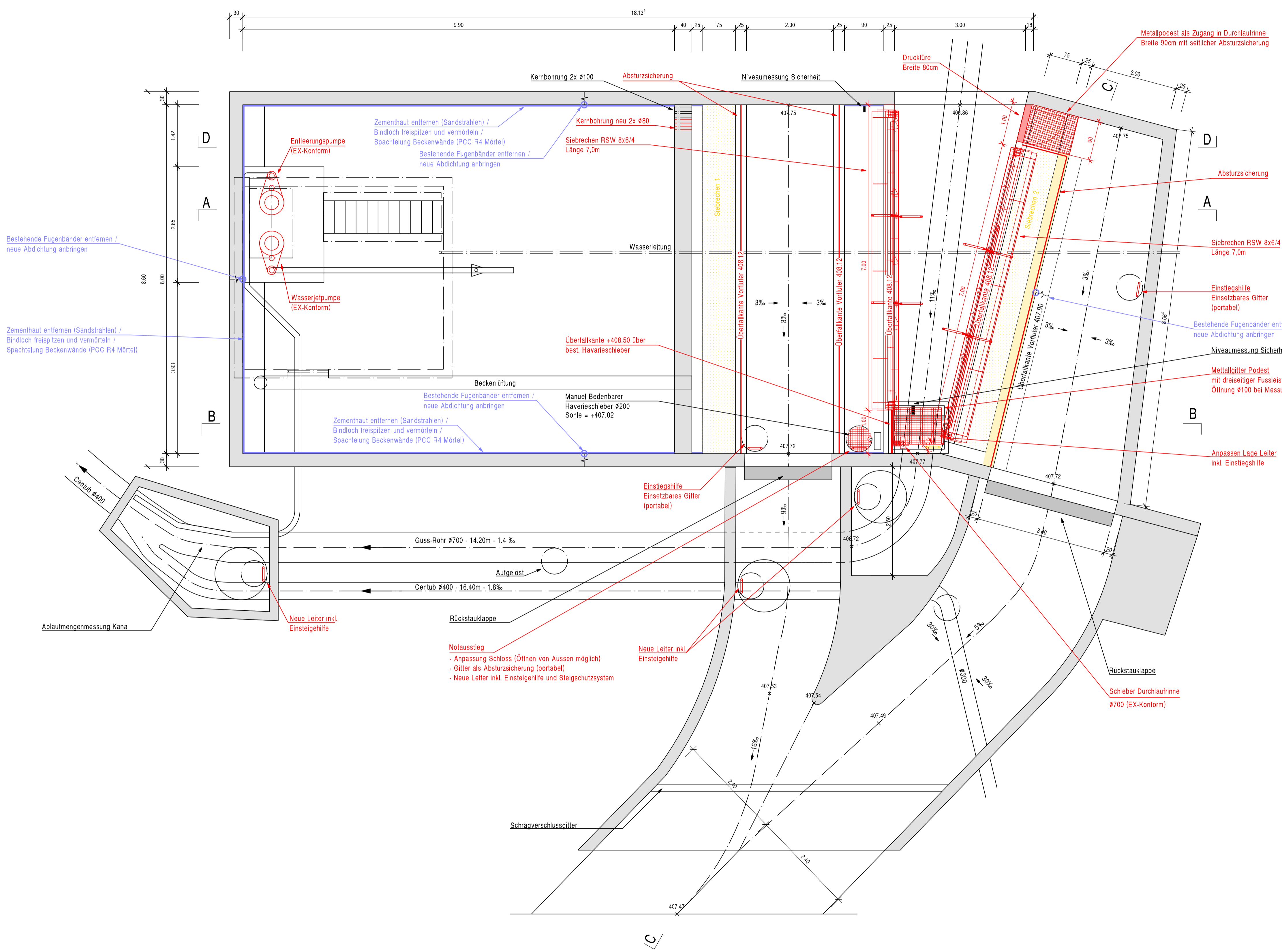
Grundriss innen 1:50
