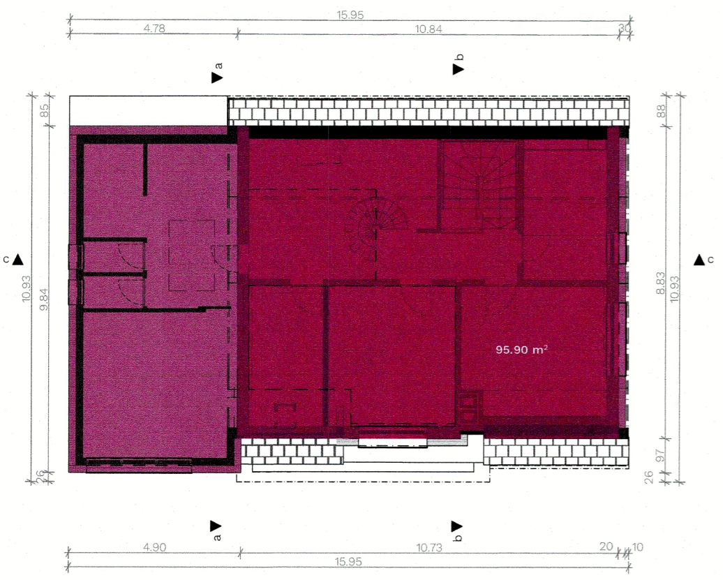
DG - Dachgeschoss
