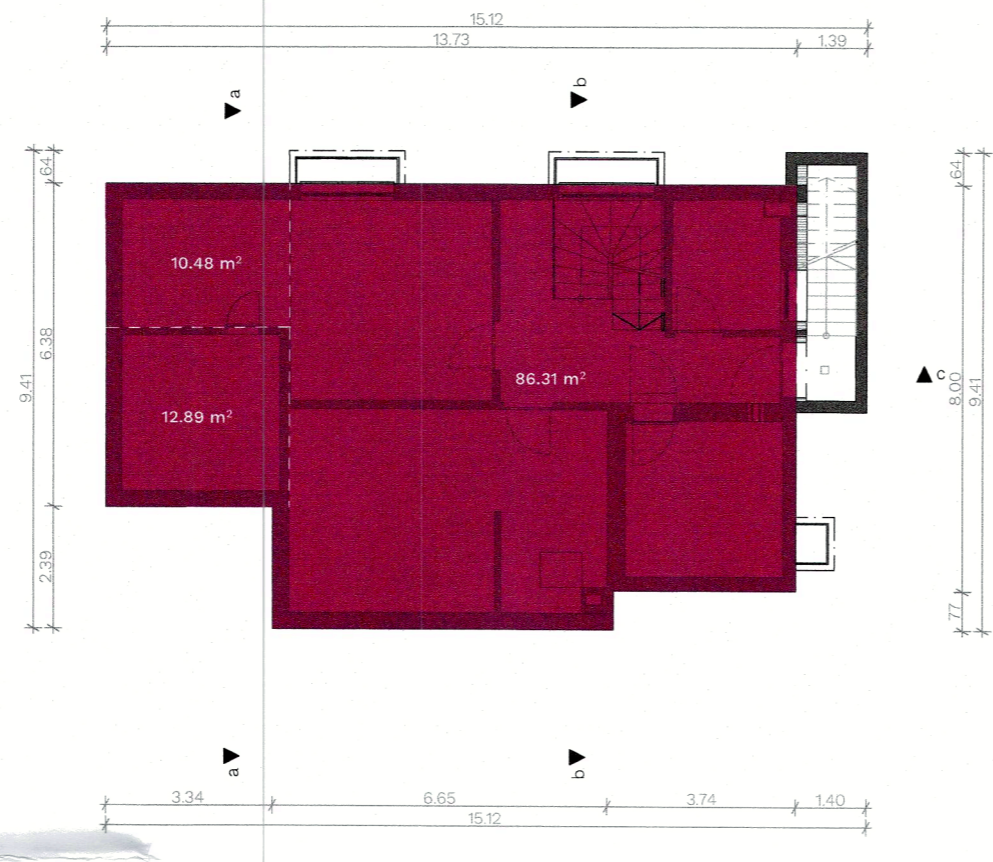
UG - Untergeschoss
