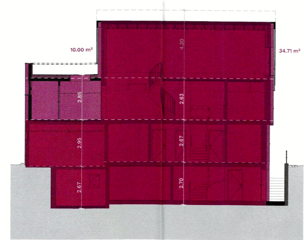
Schnitt c
