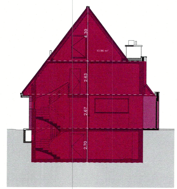
Schnitt b
