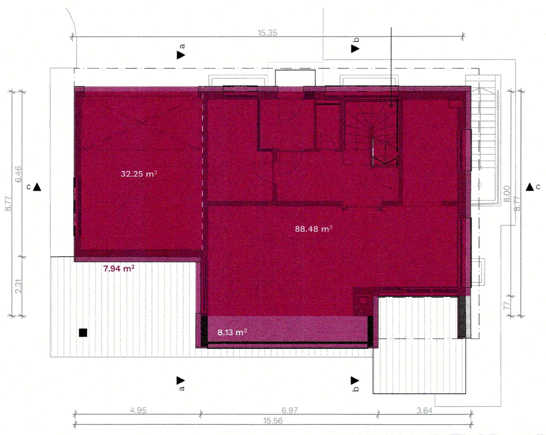
EG - Erdgeschoss
