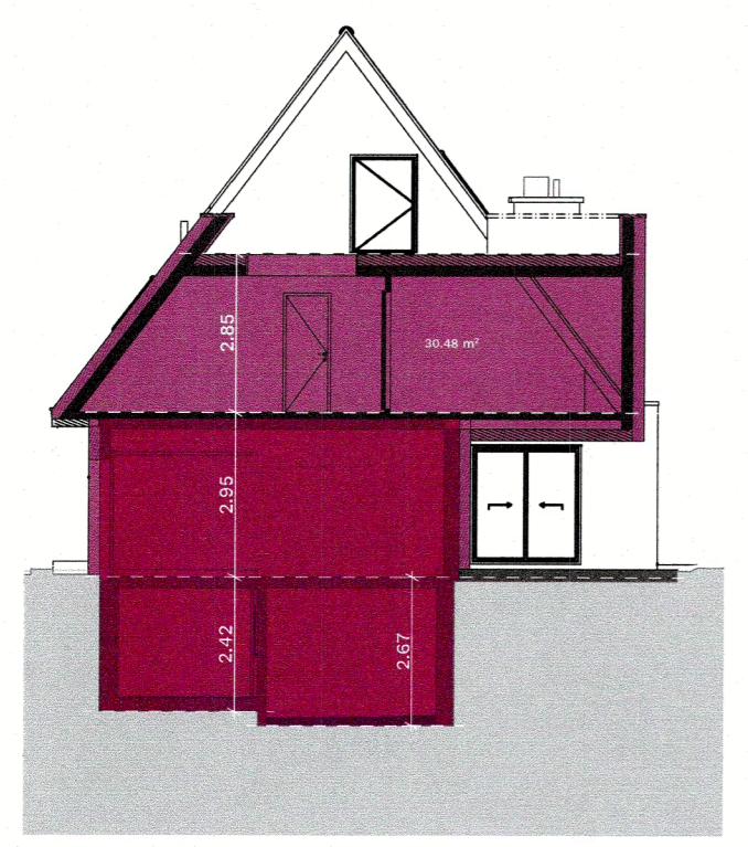
Schnitt a
