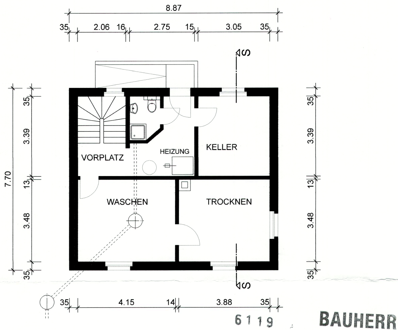
KELLERGECHOSS
