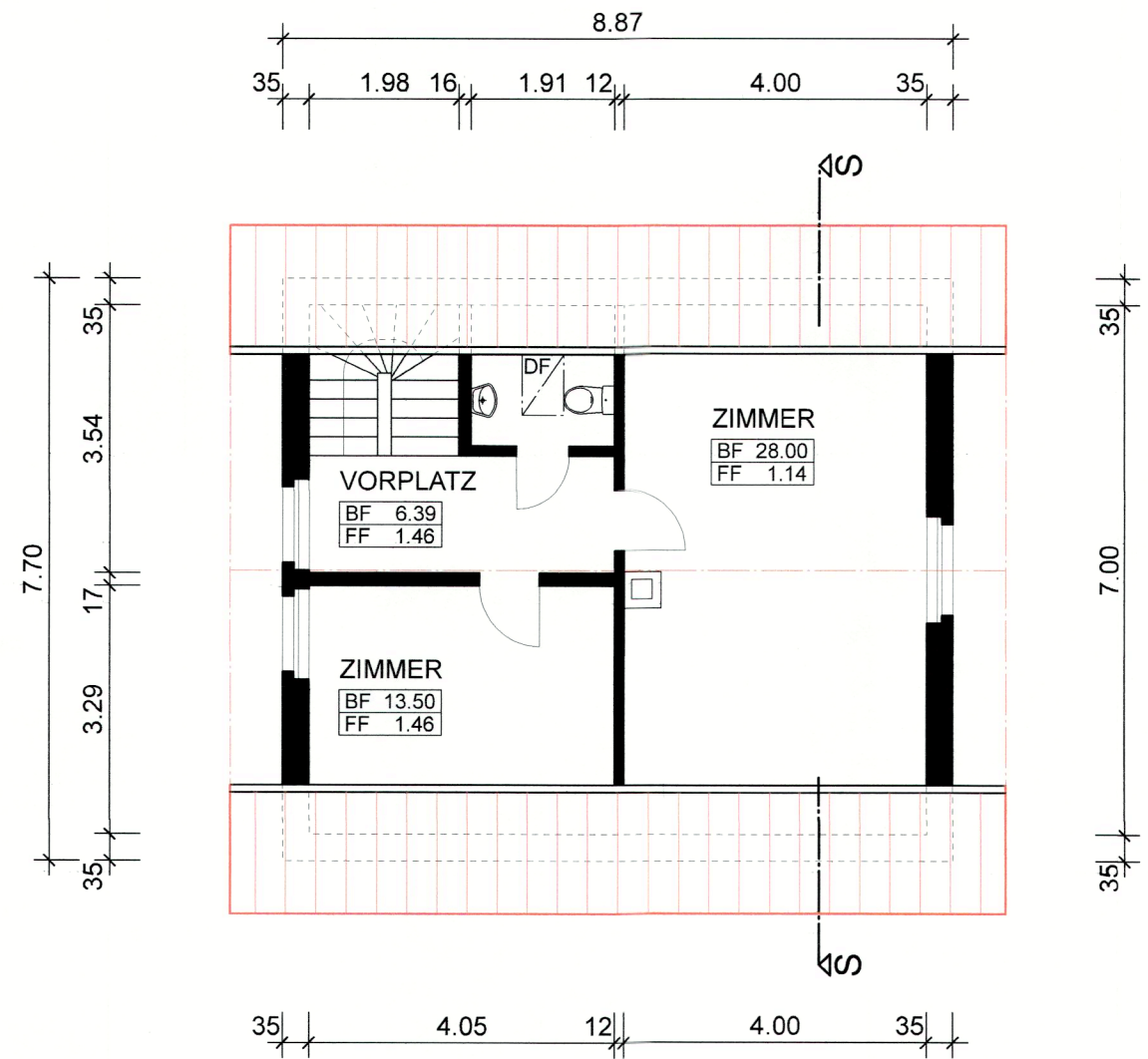
DACHGESCHOSS
