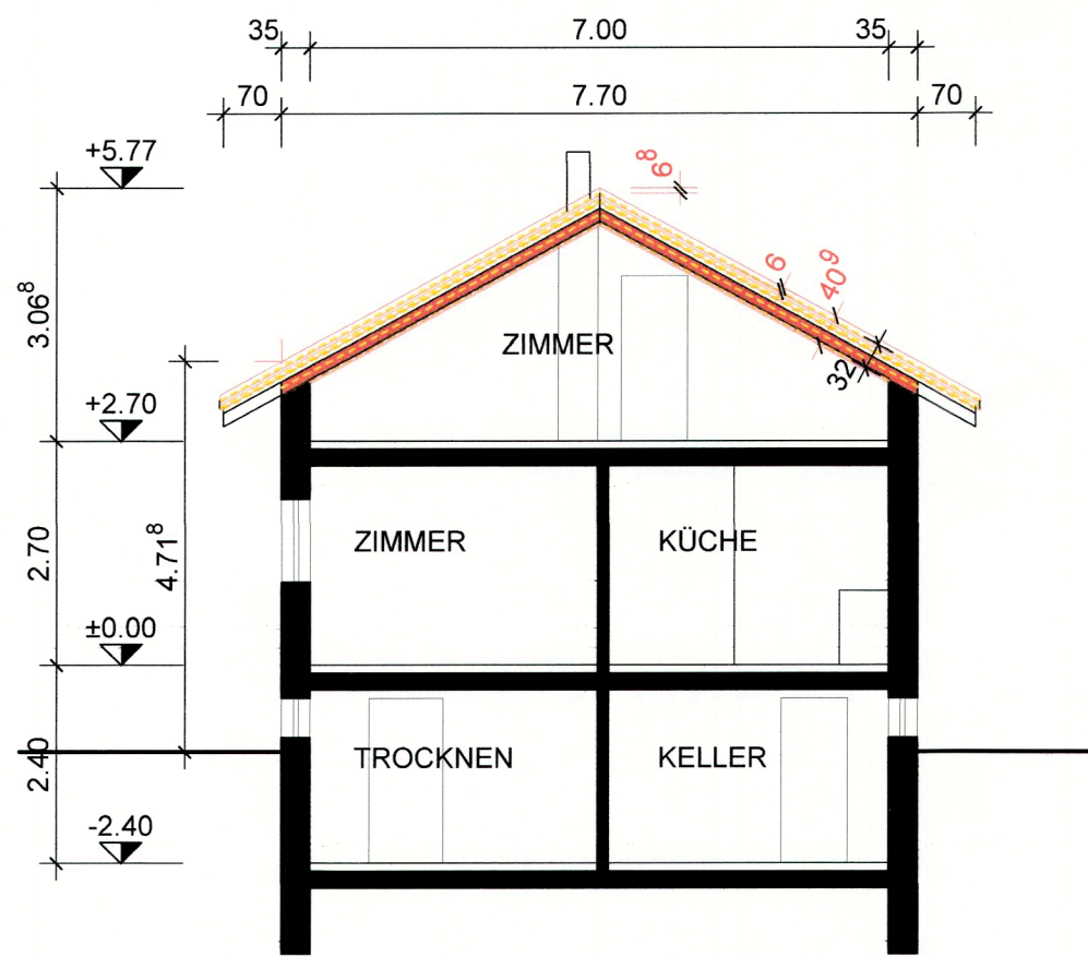
SCHNITT S-S
