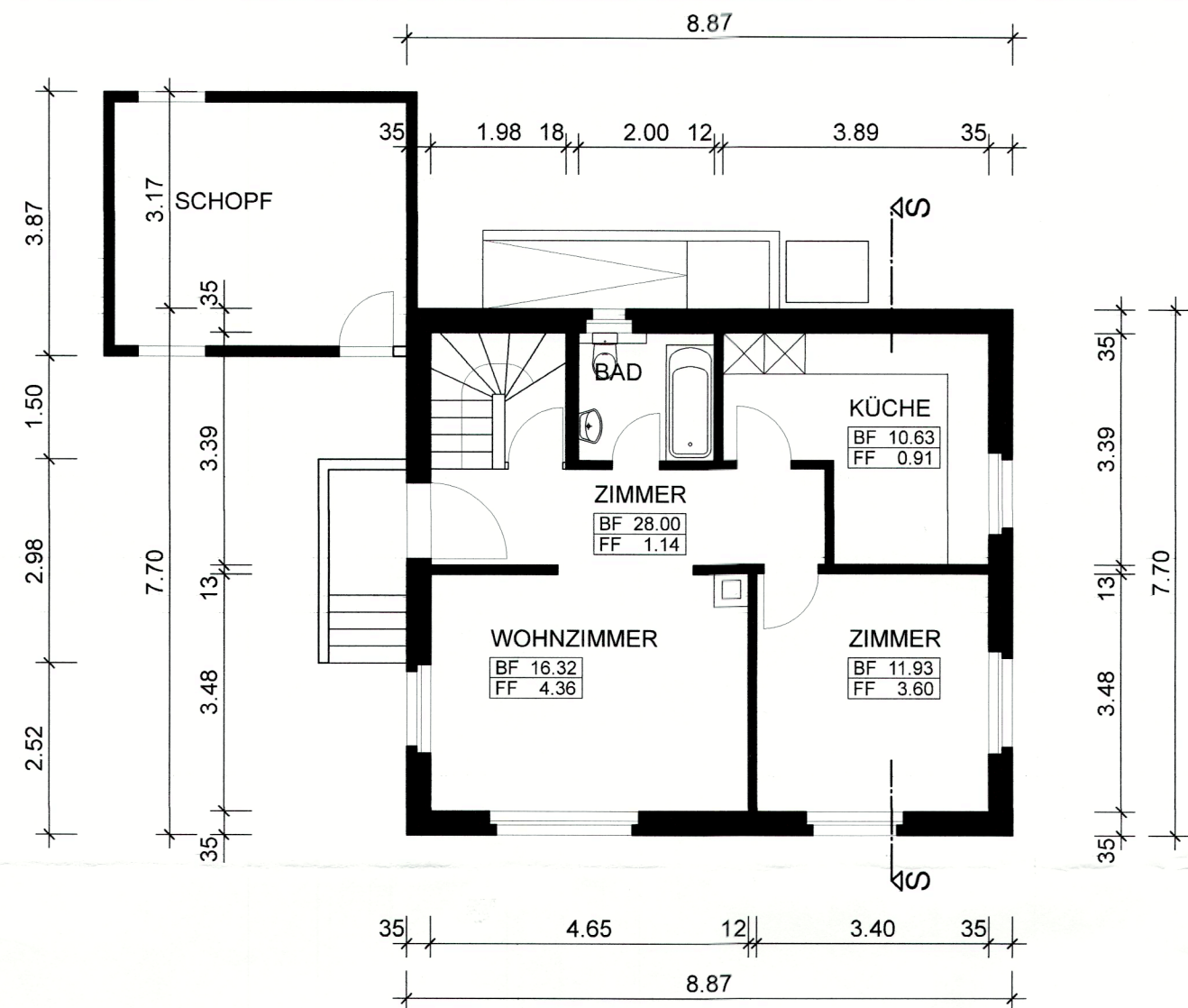
ERDGESCHOSS
