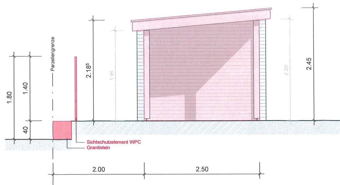
Südansicht
