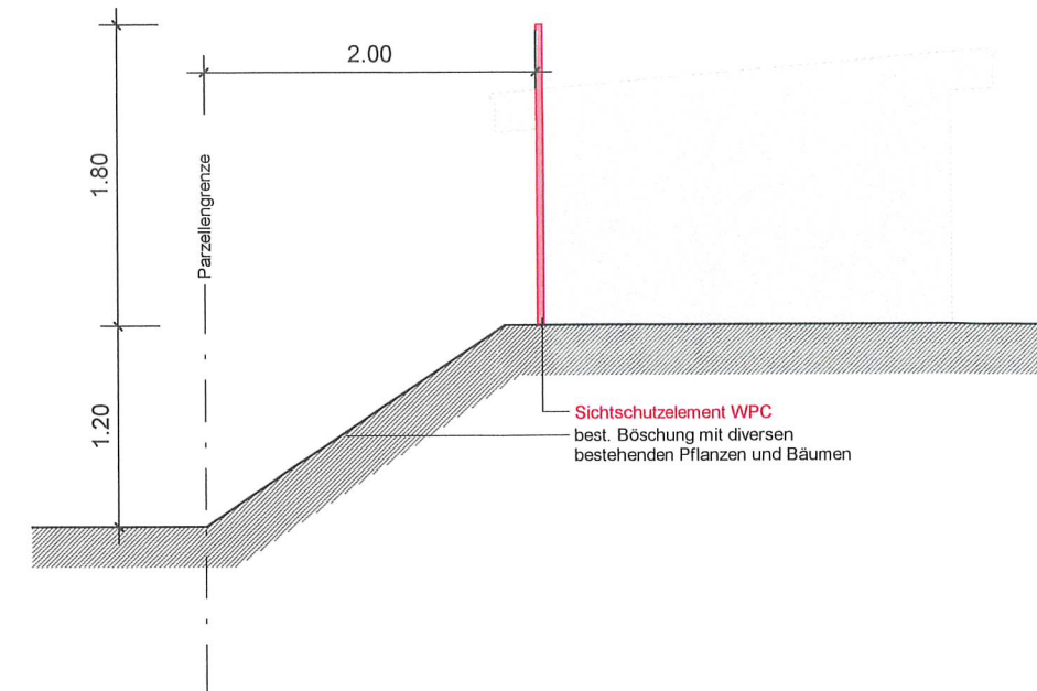
Mauerschnitt b)
