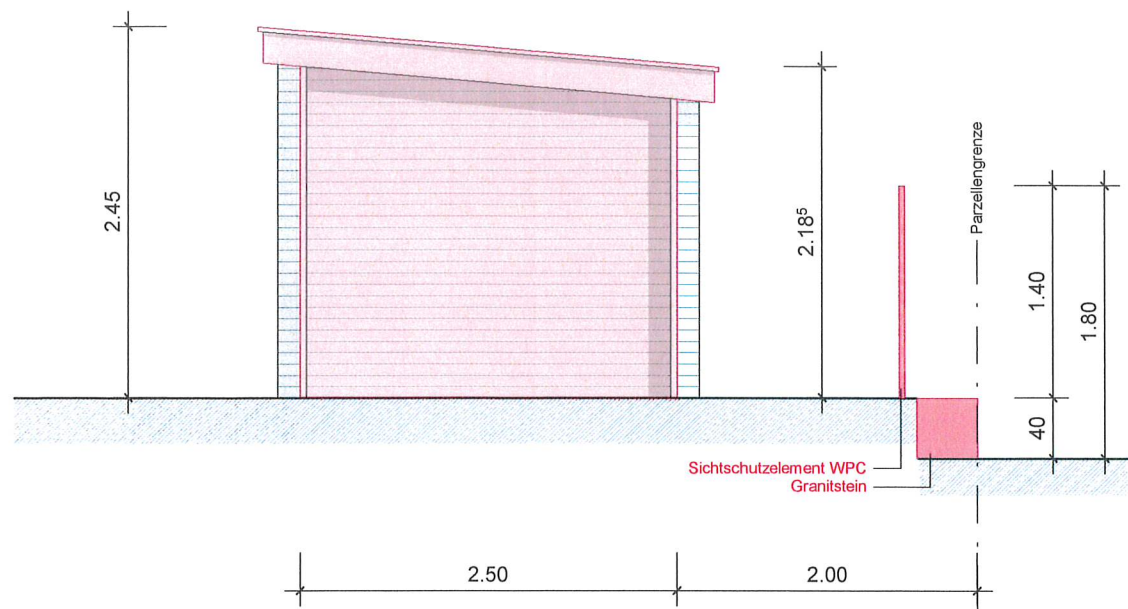
Nordansicht
